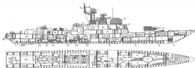
Схема общего расположения ракетного катера пр. 1224Р. 1 — фрегат; 2 — командный ракетного комплекса; 3 — цитовый катер; 4 — взрывной аппарат; 5 — ракетный комплекс; 6 — ракетный комплекс; 7 — ракетный комплекс; 8 — ракетный комплекс; 9 — ракетный комплекс; 10 — ракетный комплекс; 11 — ракетный комплекс; 12 — ракетный комплекс; 13 — ракетный комплекс; 14 — ракетный комплекс; 15 — ракетный комплекс; 16 — ракетный комплекс; 17 — ракетный комплекс; 18 — ракетный комплекс; 19 — ракетный комплекс; 20 — ракетный комплекс; 21 — ракетный комплекс; 22 — ракетный комплекс; 23 — ракетный комплекс; 24 — ракетный комплекс.
