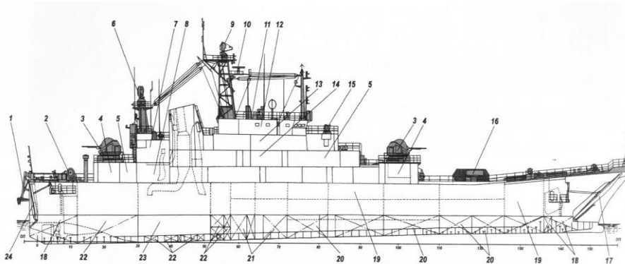
Продольный разрез БДК пр. 775 мод. I:
